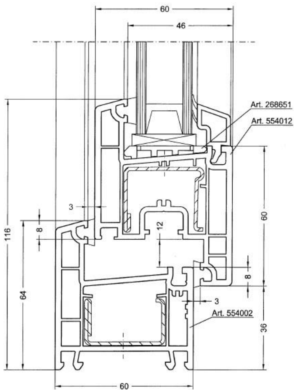
Sezione nodo Euro 60
